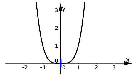
Nullstelle ohne Vorzeichenwechsel (VZW)
