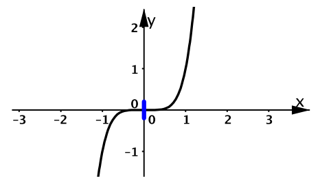
Nullstelle mit Vorzeichenwechsel (VZW)
